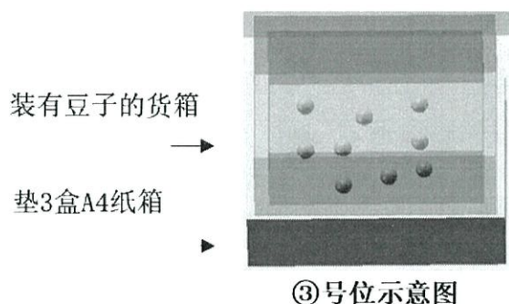
图 4 取货区置物台示意图
