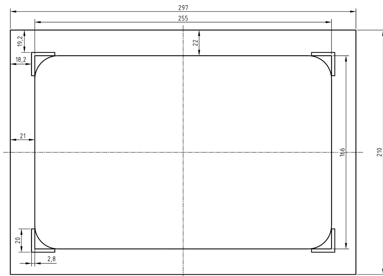
图7 L型限位器安装参考图（图示为置物台的俯视视角）
